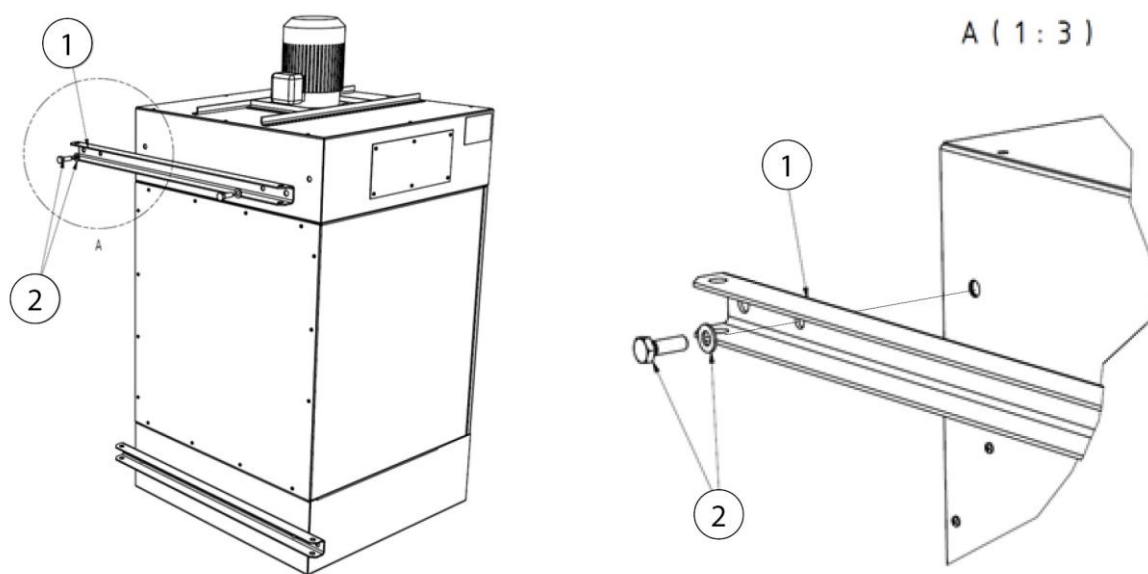
Abb. 4: Montage – Schwenk-Wandhalter
