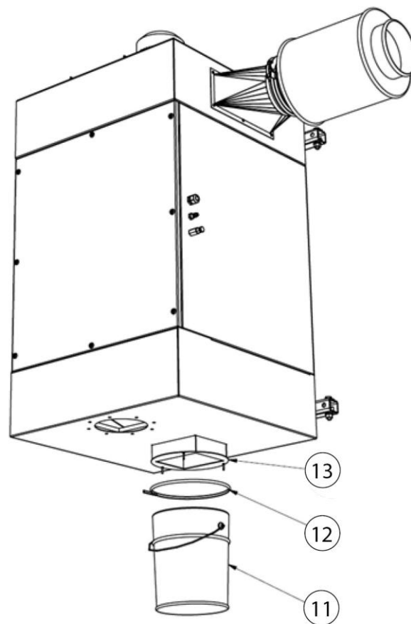
Abb. 11: Staubsammeleimer montieren
