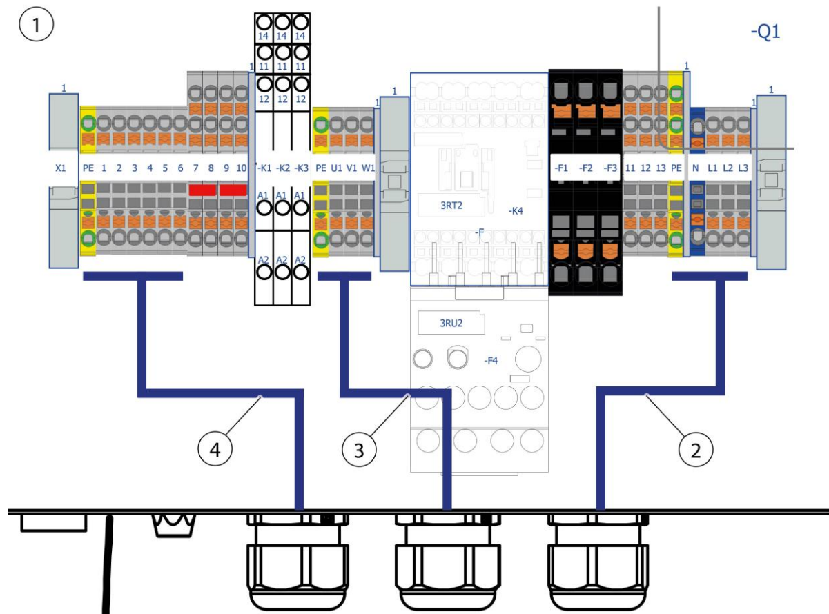
Abb. 14: Elektrischer Anschluss
