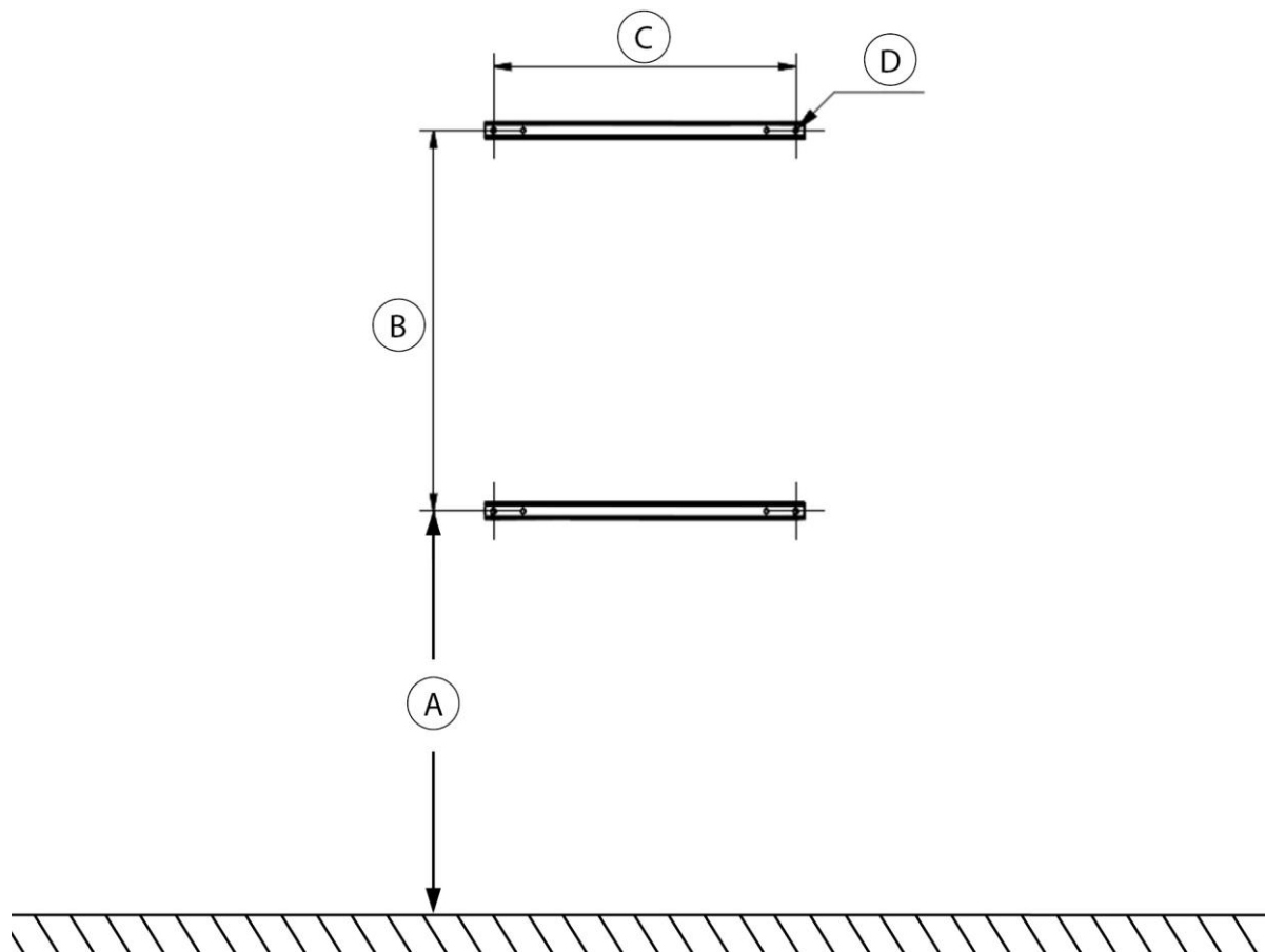
Abb. 6: Montagehöhe + Bohr-Abmessungen
