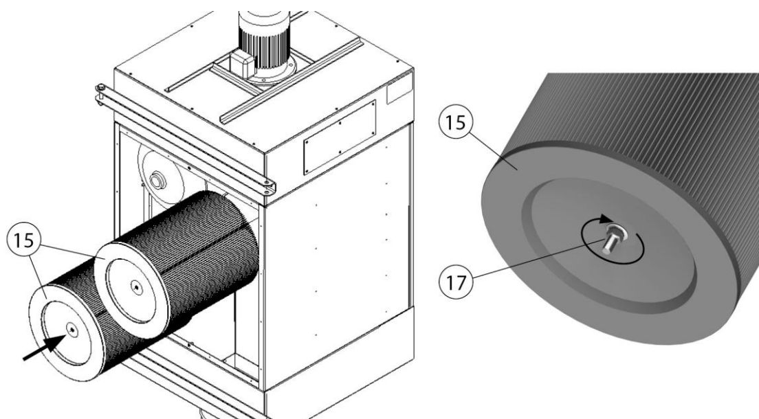
Abb. 23: Filterpatronen Einbau
